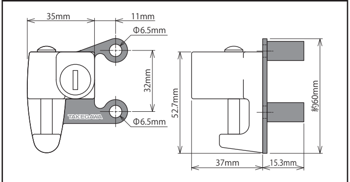
参考寸法図
