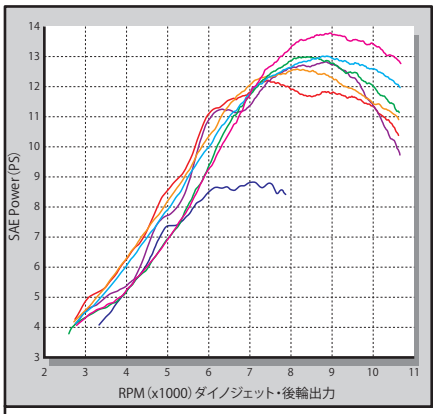
Sステージキィット145cc(カムシャフト付属) スポーツカムシャフト(N-10) FコンTYPE-X(インジェクションコントローラー) エアフィルターキィット(レッドエレメント) ビッグスロットルボディークィット Φ34
