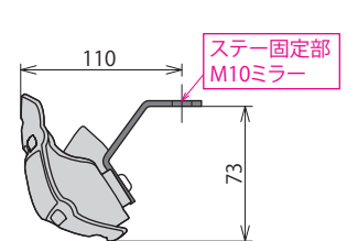
装着時の詳細図(mm)
