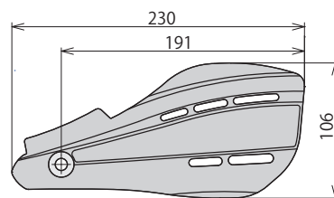
ナックルガード本体の寸法(mm)
