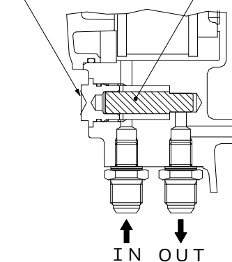
サーモスタートホールキャップ オイルホールプラグ
