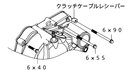
クラッチケーブルレシーバー
