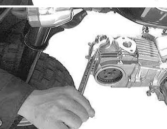
シクネスゲージ バルブシステム
