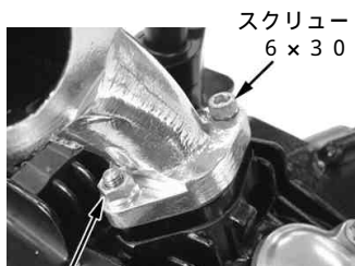
フランジナット 6mm
