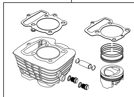
01-04-1010 Big Fin Cylinder Kit 115/124cc
