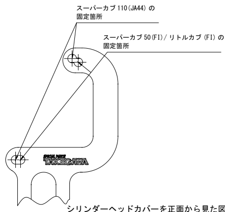
シリンダーヘッドカバーを正面から見た図
